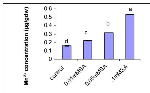
شکل ۹- اثر سالیسیلیک اسید بر جذب یون منگنز. مقادیر، میانگین سه تکرار \pm انحراف معیار بوده و مقایسه میانگین‌ها بر اساس آزمون دانکن در سطح ۵ درصد انجام شده است. حروف غیر مشترک معرف تفاوت معنی‌دار است.
