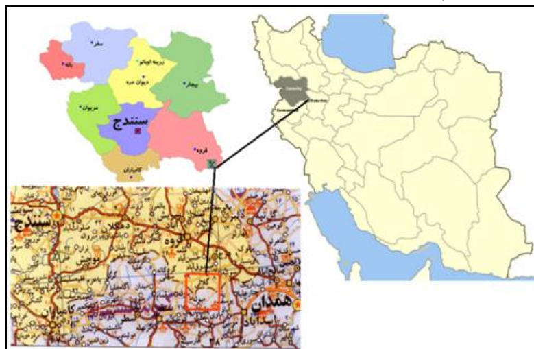
شکل ۱- نقشه موقعیت جغرافیایی محدوده مورد مطالعه (مقیاس ۱:۲۰۰۰۰۰۰۰) و راه‌های دسترسی به معدن گلالی (گلستانی، ۱۳۸۰)
