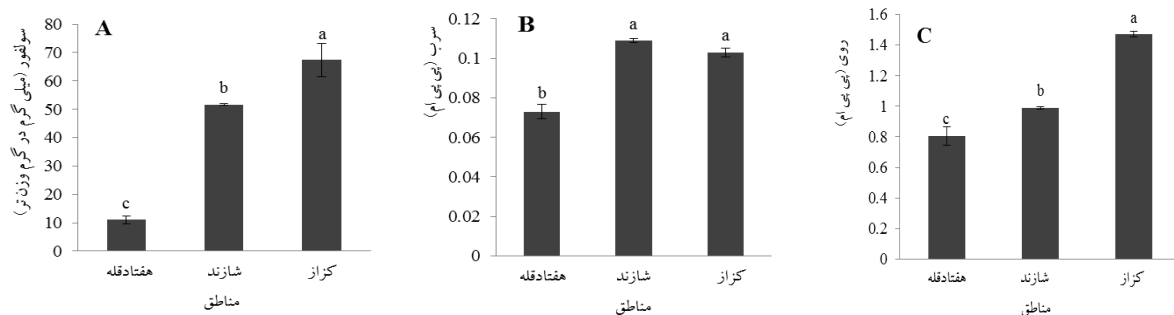
شکل ۳- تغییرات میزان گوگرد بر حسب میلی گرم بر گرم (A) وزن تر برگ، (B) عنصر سرب و (C) روی بر حسب ppm در برگ گیاه بادام در سه منطقه هفتادقله، شازند و کراز، خطوط نشان‌دهنده خطای استاندارد (SE) و حروف یکسان بیانگر عدم اختلاف معنی‌دار با استفاده از آزمون دانکن است.
