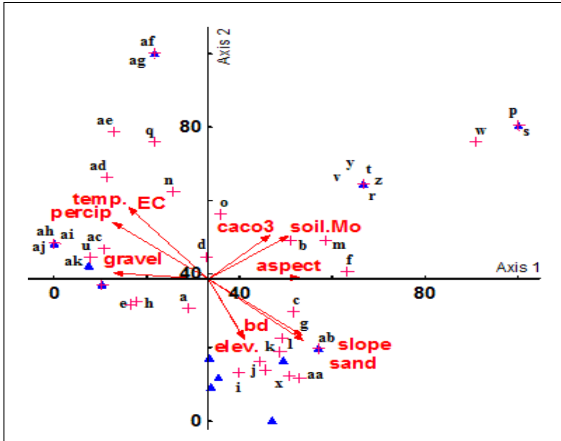
شکل ۲- نمودار پراکنش گونه‌های گیاهی مرتبط با عوامل محیطی با تحلیل تطبیقی متعارفی: EC (هدایت الکتریکی)، pH (اسیدیته)، sand (درصد سیلت)، silt (درصد رس)، clay (درصد کربن آلی)، oc (درصد آهنک)، CaCO 3 (درصد آهک)، Soil.Mo (درصد رطوبت اشباع)، Soil.Mo (درصد شن)، soil.Mo (رطوبت خاک)، prosity (تخلخل)، gravel (سنگ‌ریزه)، bd (وزن مخصوص ظاهری)، slope (شیب)، elev (ارتفاع از سطح دریا)، temp (درجه حرارت)، percip (بارش)، aspect (جهت شیب)، مثلث آبی (مکان پراکنش)، فلش (شاخص محیطی)، + (گونه‌های گیاهی)، a ( Ephedra procera )، b ( Centaurea virgata )، c ( Bromus tectorum )، d ( Annual forbs )، e محیطی، j ( Achillea )، i ( Festuca pinifolia )، h ( Agropyrom trichophorum )، g ( Stipa barbata )، f ( Poa bulbosa )، n ( Alyssum )، m ( Acanthophyllum heterophyllum )، l ( Ziziphora persica )، k ( Prangos latiloba )، j ( millefolium )، r ( Achillea )، s ( Secale montanum )، q ( Noea mucronata )، p ( Echinops aucheri )، o ( Cousinia atropatana )، x ( bracteatum )، w ( Ceratocarpus arenarius )، v ( Centaurea glastifolia )، u ( Hordeum glaucum )، t ( Melica persica )، y ( millefolium )، ab ( Acanthophyllum heterophyllum )، aa ( Bromus brizifomis )، z ( Lepidium perfoliatum )، y ( Anthemis atropatana )، ag ( Cirsium arvense )، af ( Medicago radiata )، ae ( Annual grasses )، ad ( Anthemis atropatana )، ac ( Poa annua )، ak ( Centaurea persica )، aj ( Anchusa iranica )، ai ( Pteropyron aucheri )، ah ( Fumaria parviflora )، ( Kochia scoparia )
